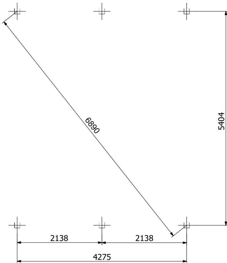
B-B ( 1 : 60 )
