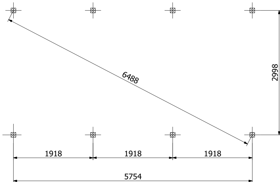
A-A ( 1 : 55 )
